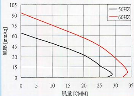
TBO-321010 [入口10"出口10"]
