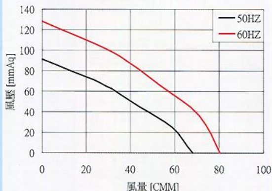
TBO-401010 [入口10"出口10"]
