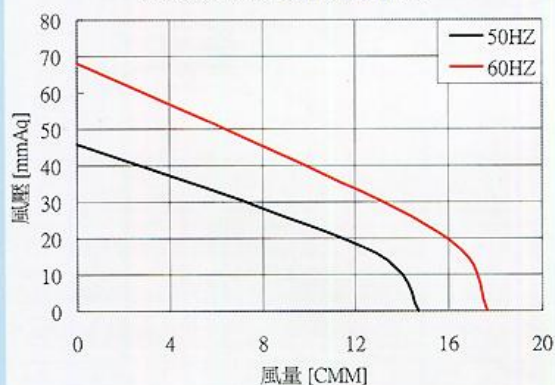
TBO-270606 [入口6"出口6"]
