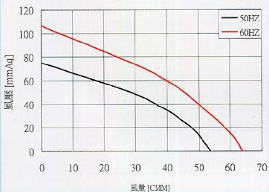
TBO-371212 [入口12"出口12"]
