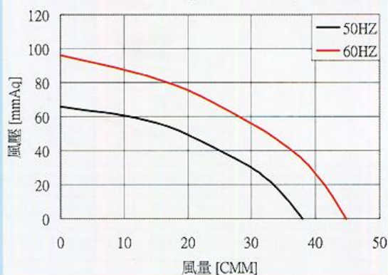
TBO-350808 [入口8"出口8"]
