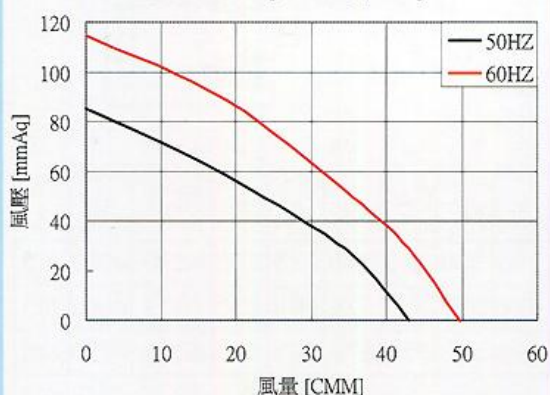
TBO-370808 [入口8"出口8"]
